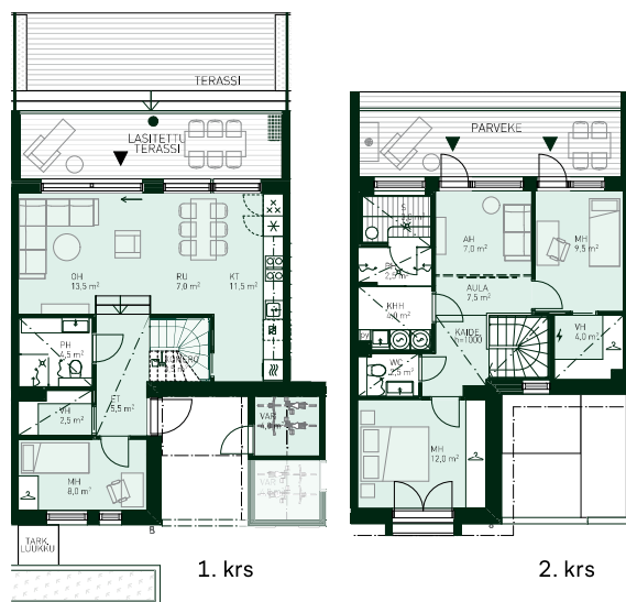
A04-huoneistopohja
