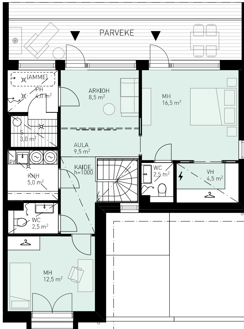
2. kerros
