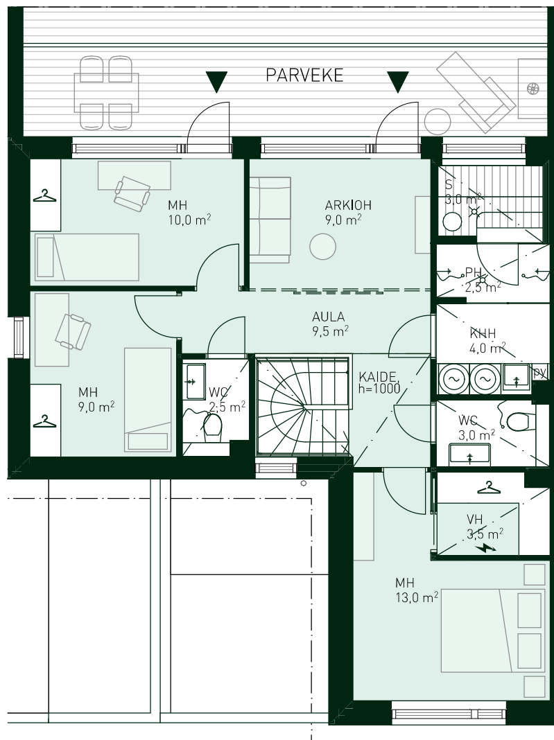
2. kerros
