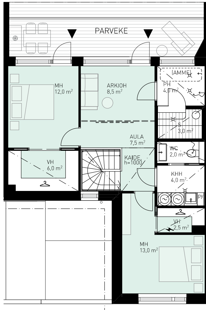
2. kerros
