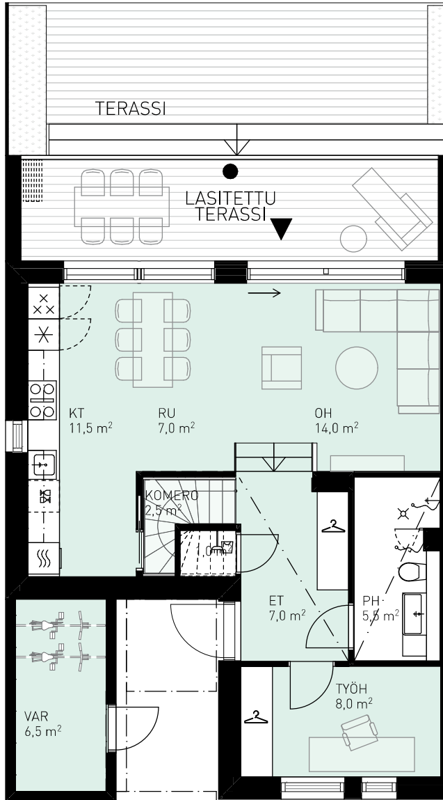
1. kerros
