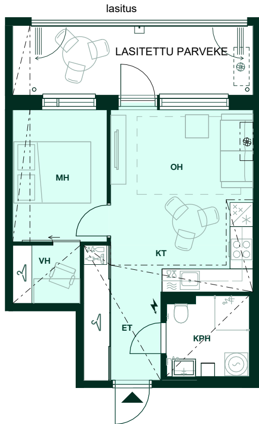
VAIHTOEHTOPOHJA 1
